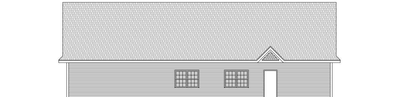
SW ELEVATION
